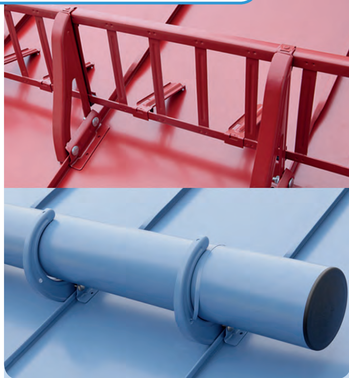
Blickfang auf dem Blechdach: Farbbeschichtete Schneefangbalken und Schneefanggitter
