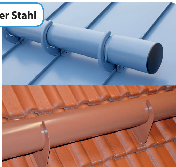
Schneefangbalken aus Aluminium oder verzinktem Stahl, beschichtet in der Farbe des Blech- oder Ziegeldachs.
